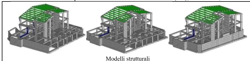
Modelli strutturali
